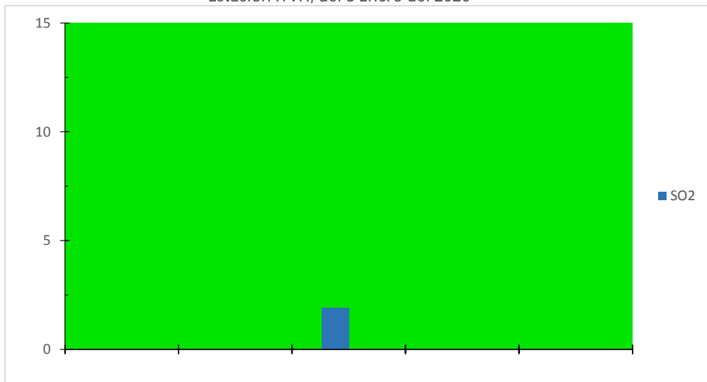
Gráfica de IMECAS de Dioxido de azufre ( SO_2 ) en la ciudad de Villahermosa, Tabasco. Estación ITVH, del 8 Enero del 2020
