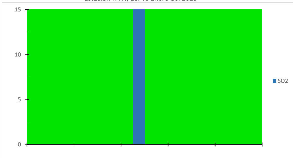
Gráfica de IMECAS de Dioxido de azufre ( SO_2 ) en la ciudad de Villahermosa, Tabasco. Estación ITVH, del 15 Enero del 2020
