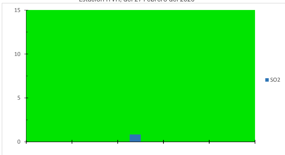
Gráfica de IMECAS de Dioxido de azufre (SO 2 ) en la ciudad de Villahermosa, Tabasco. Estación ITVH, del 27 Febrero del 2020
