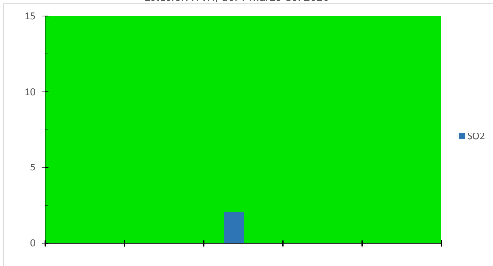
Gráfica de IMECAS de Dioxido de azufre ( SO_2 ) en la ciudad de Villahermosa, Tabasco. Estación ITVH, del 9 Marzo del 2020
