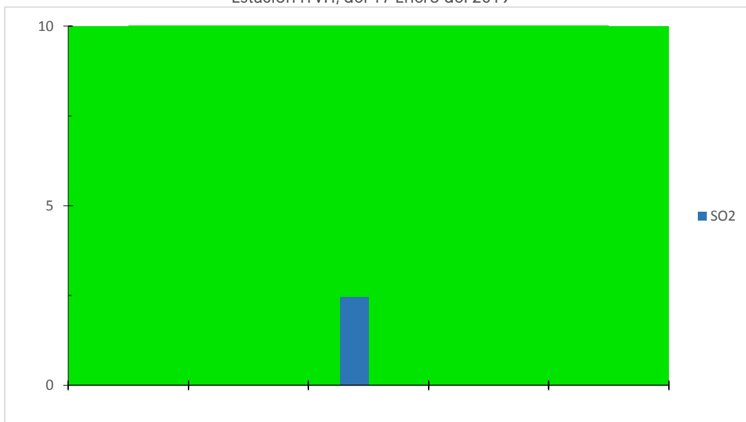
Gráfica de IMECAS de Dioxido de azufre ( SO_2 ) en la ciudad de Villahermosa, Tabasco. Estación ITVH, del 17 Enero del 2019
