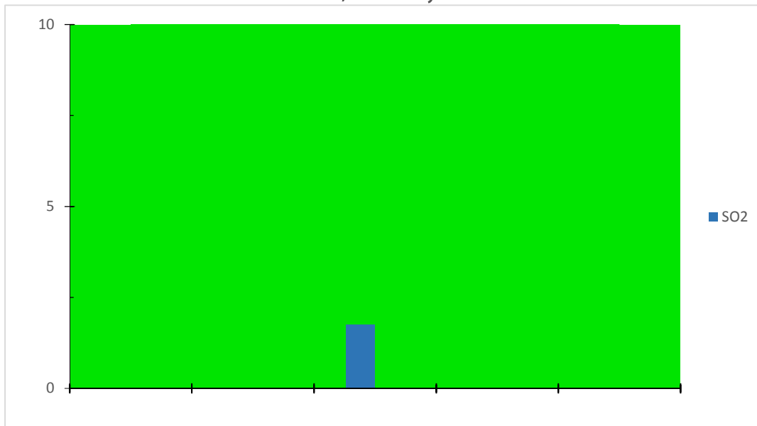
Gráfica de IMECAS de Dioxido de azufre (SO 2 ) en la ciudad de Villahermosa, Tabasco. Estación ITVH, del 27 Mayo del 2019
