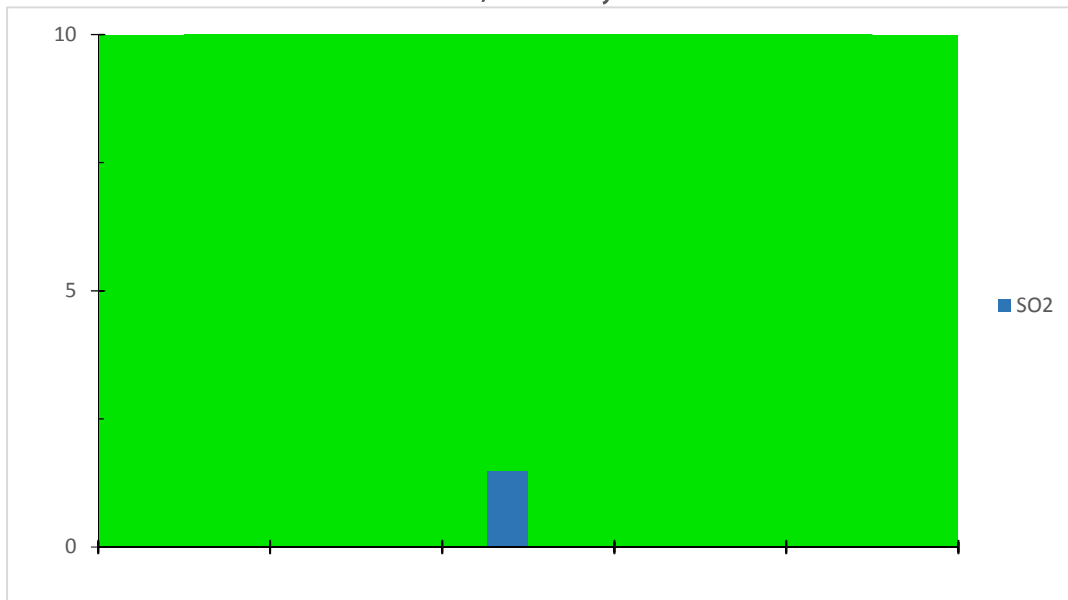
Gráfica de IMECAS de Dioxido de azufre ( SO_2 ) en la ciudad de Villahermosa, Tabasco. Estación ITVH, del 30 Mayo del 2019
