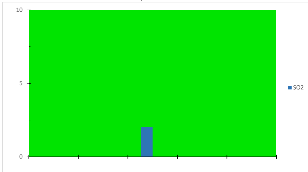
Gráfica de IMECAS de Dioxido de azufre (SO 2 ) en la ciudad de Villahermosa, Tabasco. Estación ITVH, del 5 Junio del 2019
