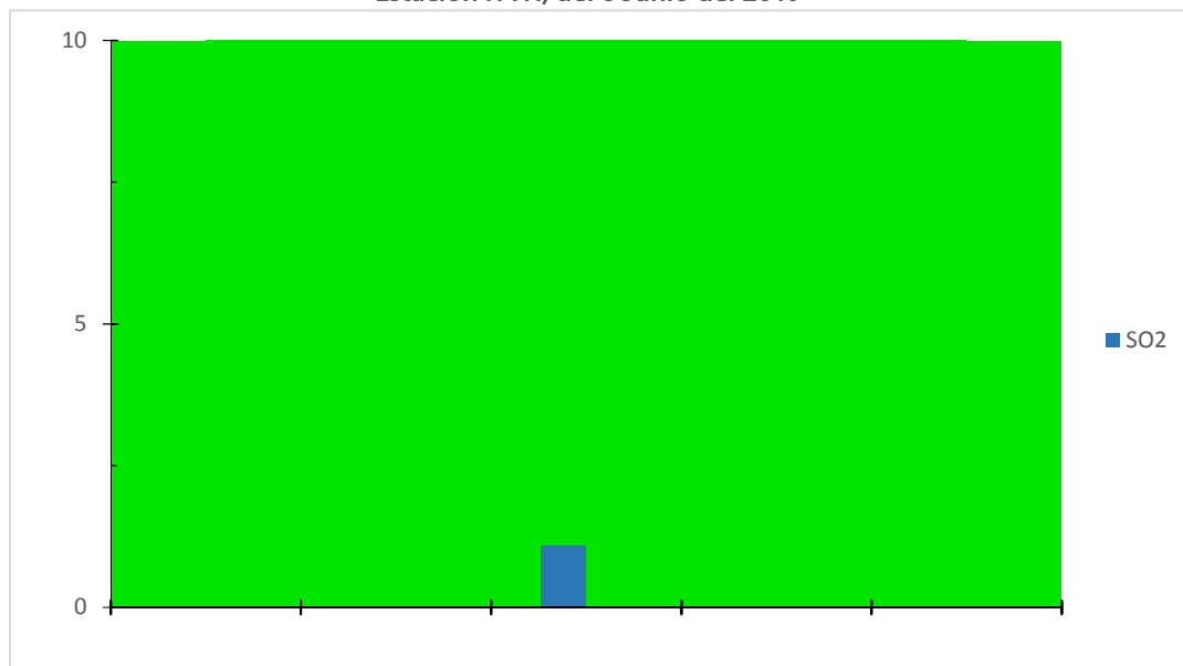
Gráfica de IMECAS de Dioxido de azufre (SO 2 ) en la ciudad de Villahermosa, Tabasco. Estación ITVH, del 6 Junio del 2019
