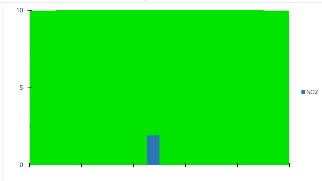
Gráfica de IMECAS de Dioxido de azufre (SO 2 ) en la ciudad de Villahermosa, Tabasco. Estación ITVH, del 10 Junio del 2019
