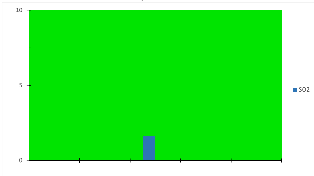
Gráfica de IMECAS de Dioxido de azufre ( SO_2 ) en la ciudad de Villahermosa, Tabasco. Estación ITVH, del 11 Junio del 2019
