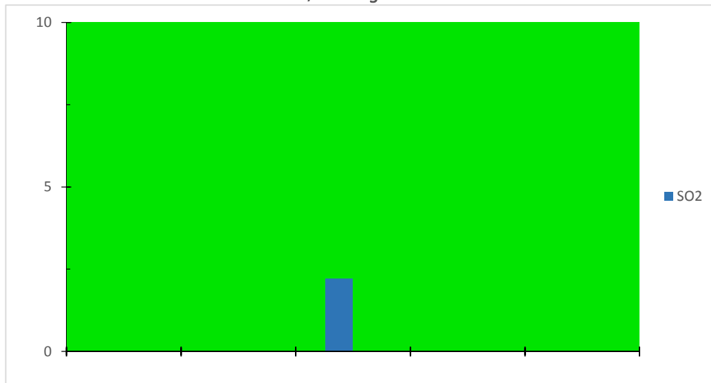
Gráfica de IMECAS de Dioxido de azufre (SO 2 ) en la ciudad de Villahermosa, Tabasco. Estación ITVH, del 1 Agosto del 2019
