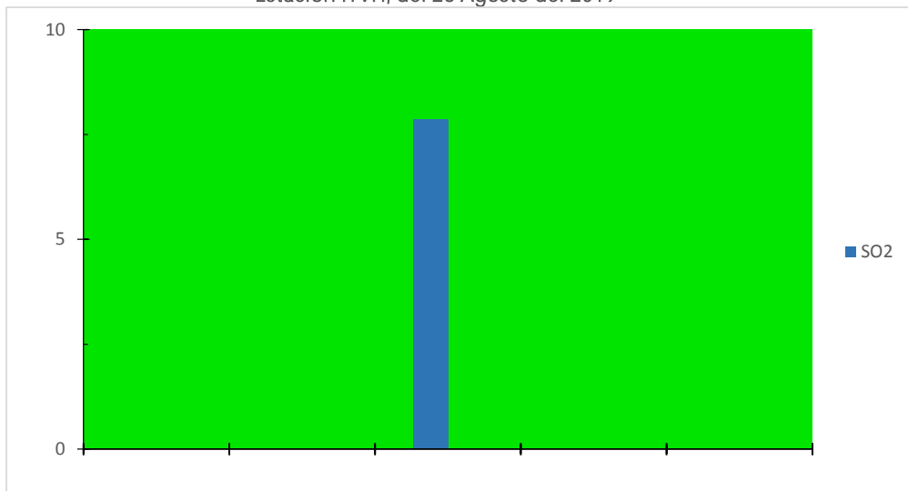
Gráfica de IMECAS de Dioxido de azufre ( SO_2 ) en la ciudad de Villahermosa, Tabasco. Estación ITVH, del 26 Agosto del 2019
