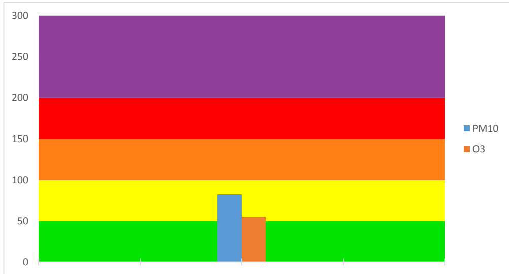
Gráfica de IMECAS de Ozono ( O_3 ) y Partículas ( PM_{10} ); en la ciudad de Villahermosa, Tabasco. Estación ITVH, del 26 Agosto del 2019
