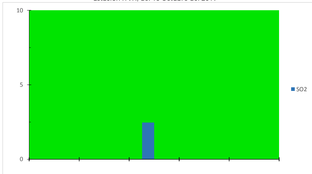
Gráfica de IMECAS de Dioxido de azufre ( SO_2 ) en la ciudad de Villahermosa, Tabasco. Estación ITVH, del 15 Octubre del 2019
