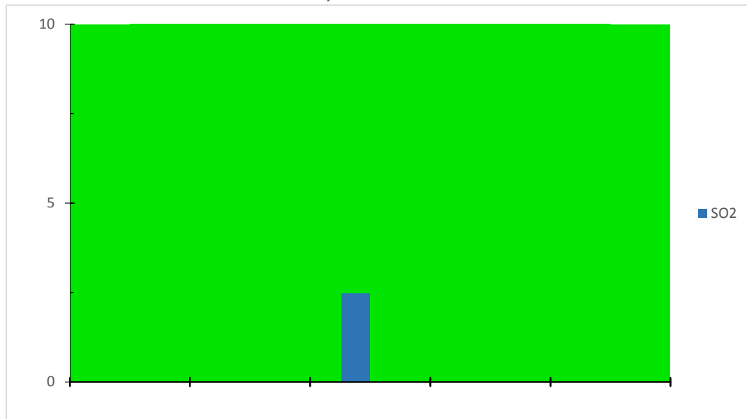
Gráfica de IMECAS de Dioxido de azufre (SO 2 ) en la ciudad de Villahermosa, Tabasco. Estación ITVH, del 22 Octubre del 2019
