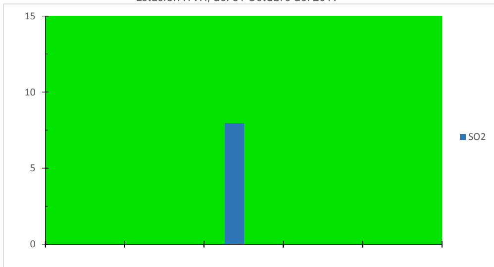
Gráfica de IMECAS de Dioxido de azufre ( SO_2 ) en la ciudad de Villahermosa, Tabasco. Estación ITVH, del 31 Octubre del 2019
