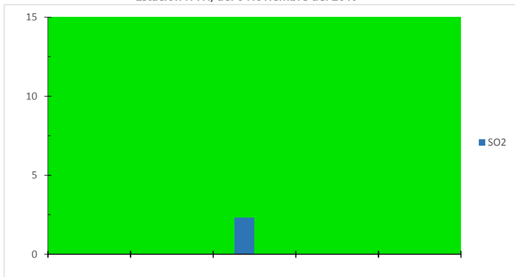
Gráfica de IMECAS de Dioxido de azufre ( SO_2 ) en la ciudad de Villahermosa, Tabasco. Estación ITVH, del 6 Noviembre del 2019
