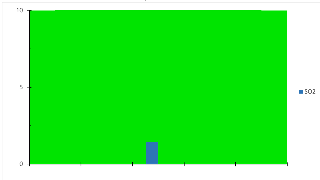
Gráfica de IMECAS de Dioxido de azufre (SO 2 ) en la ciudad de Villahermosa, Tabasco. Estación ITVH, del 15 Abril del 2019
