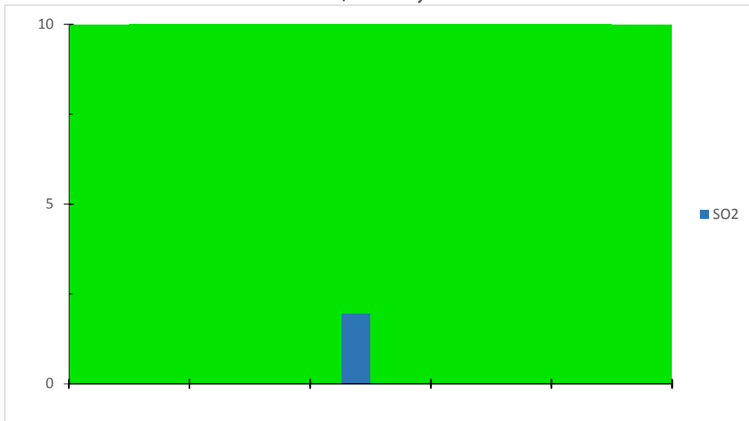
Gráfica de IMECAS de Dioxido de azufre (SO 2 ) en la ciudad de Villahermosa, Tabasco. Estación ITVH, del 2 Mayo del 2019
