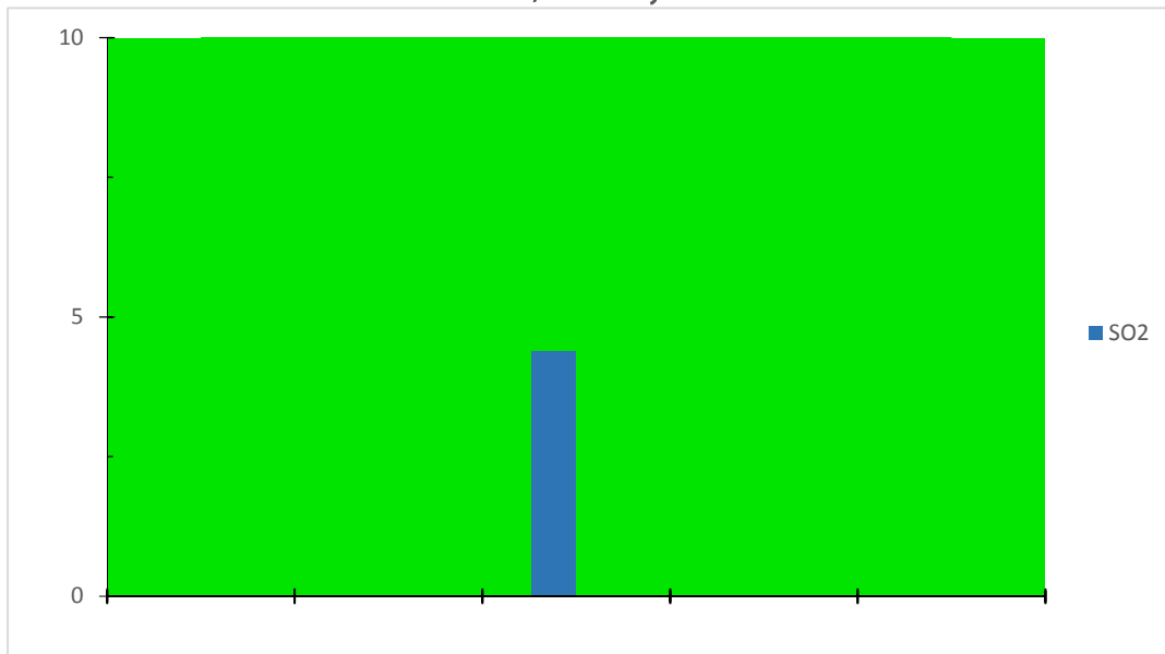
Gráfica de IMECAS de Dioxido de azufre (SO 2 ) en la ciudad de Villahermosa, Tabasco. Estación ITVH, del 7 Mayo del 2019
