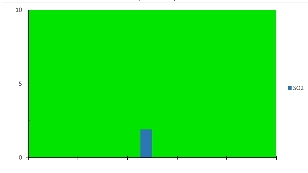
Gráfica de IMECAS de Dioxido de azufre ( SO_2 ) en la ciudad de Villahermosa, Tabasco. Estación ITVH, del 20 Mayo del 2019
